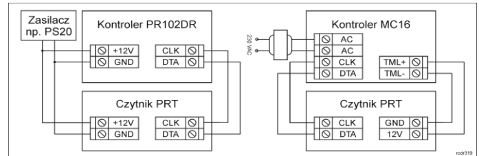
Rys. 4 Podłączenie czytnika do przykładowego kontrolera systemu RACS 4 (PR102DR) i kontrolera systemu RACS 5 (MC16) - praca terminalowa
